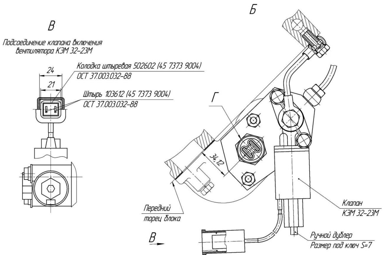
Рисунок 2 – Подключение КЭМ
