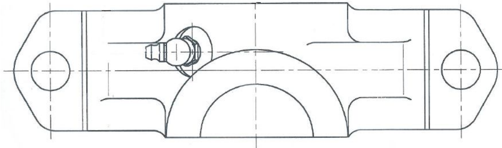
Рис.1 Хомут кронштейна передней опоры 238НД5-1001010 вид сверху.
