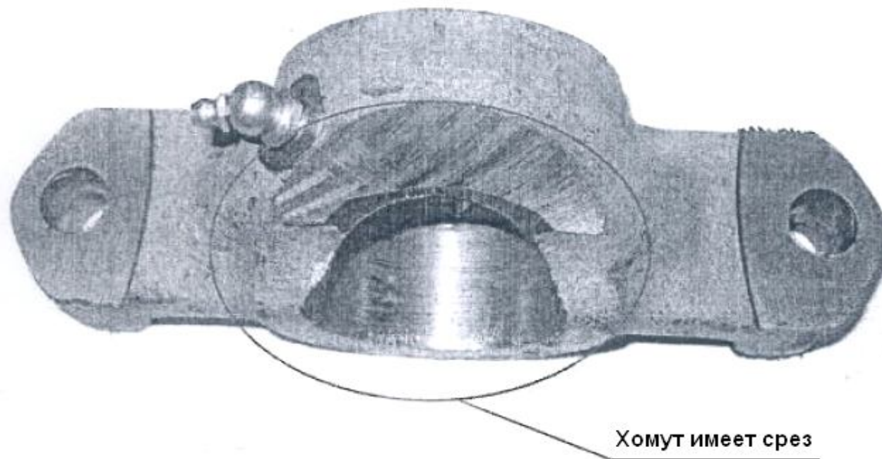
Фото 1. Хомут кронштейна передней опоры 238НД5-1001010
