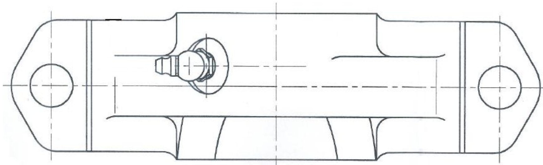
Рис. 2 Хомут кронштейна передней опоры 238НБ-1001010 вид сверху.
