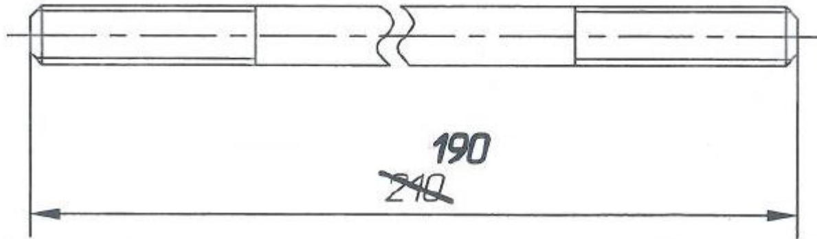
Рис.1 Тяга рычага управления регулятором 850.1108051.
