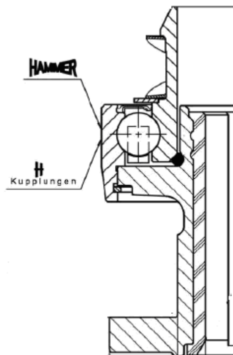
Рис. 3 Муфта выключения сцепления.
