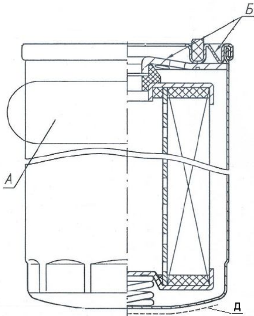
Рис. 2. Фильтр сменный «DIFA 6103» для топлива.
