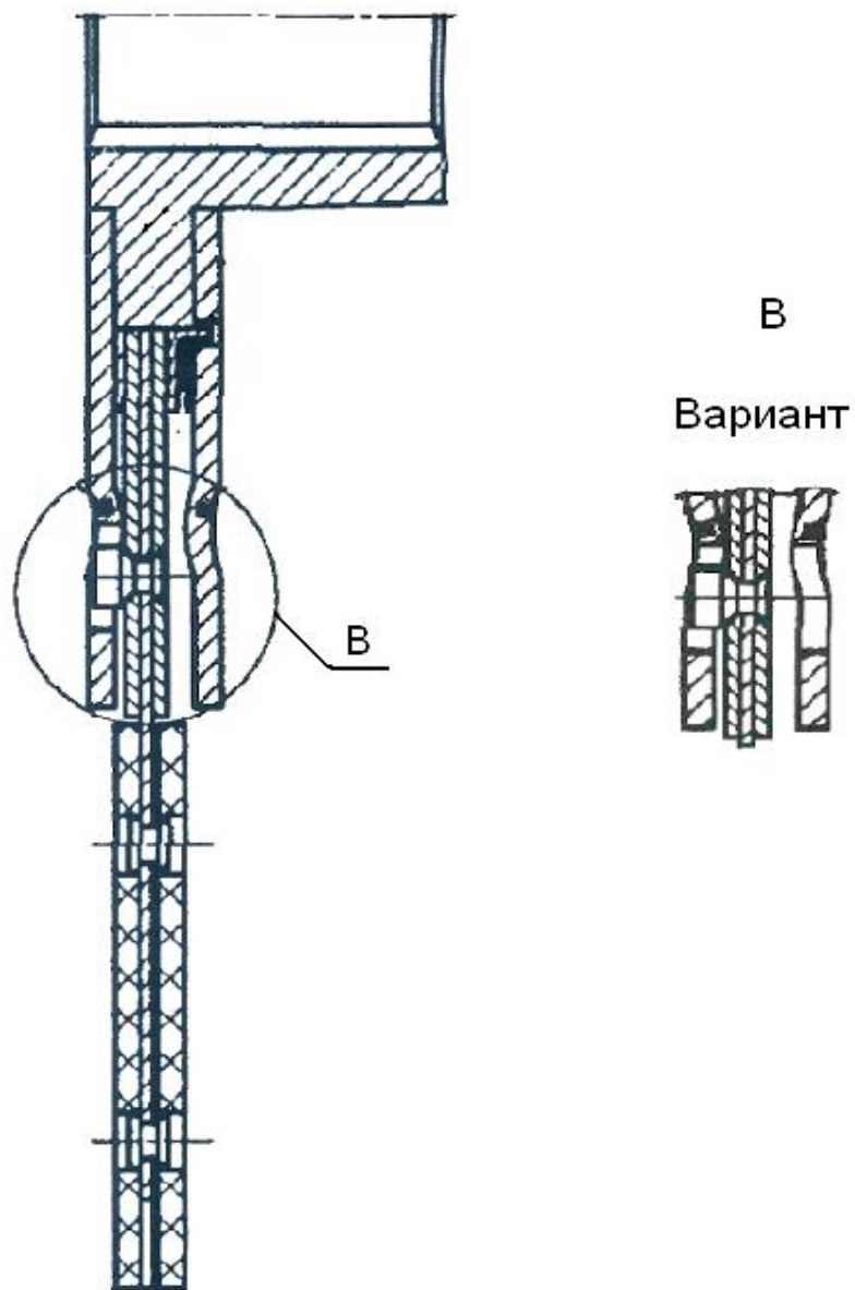
Рис. 2 Вариант исполнения диска сцепления ведомого производства ООО «СМТ авто»
