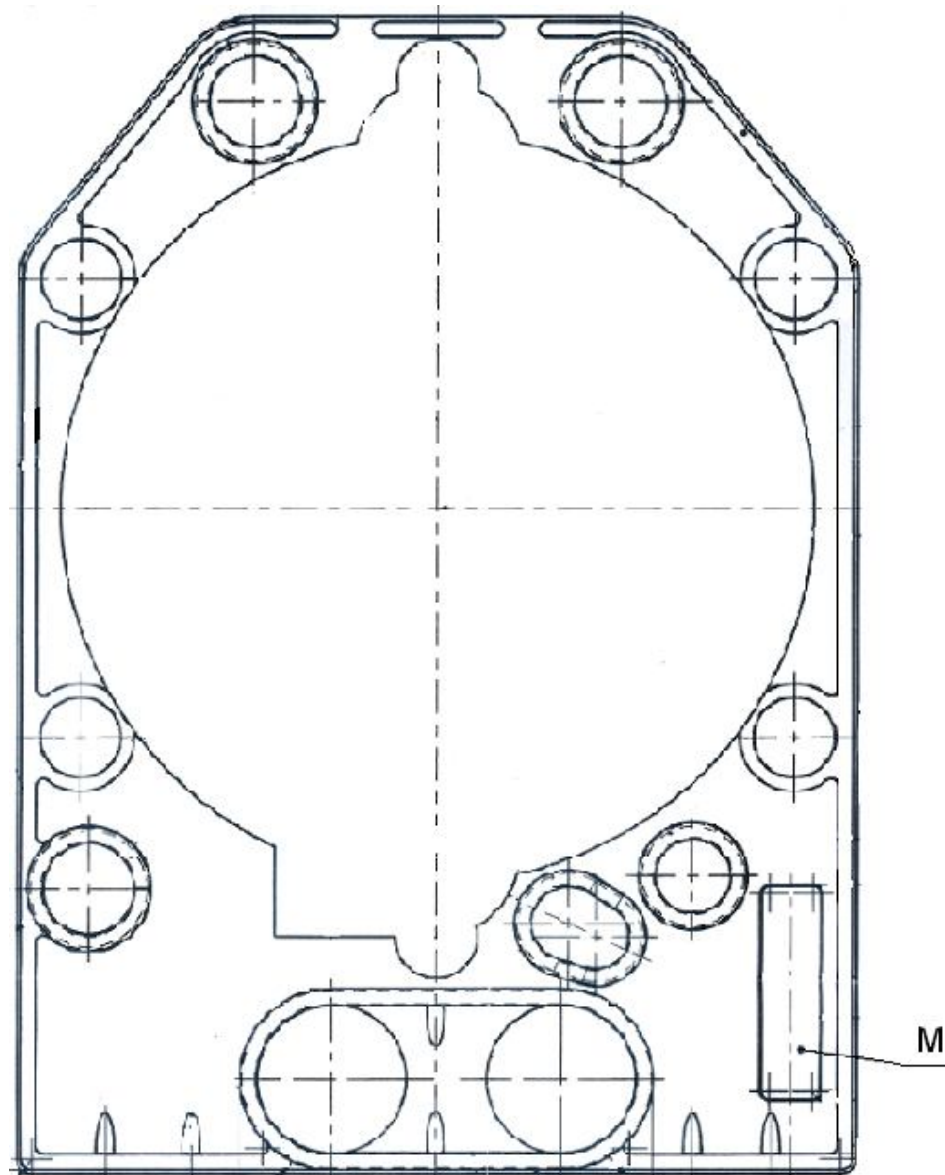
Рис. 1 Прокладка уплотнительная головки цилиндра 840.1003213-03 .
