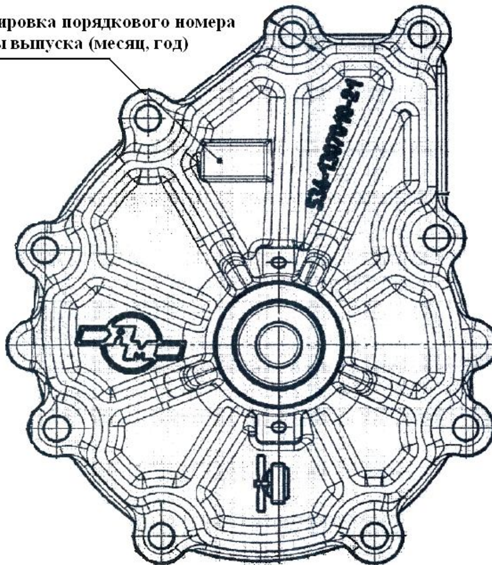
Рис. 1. Водяной насос 536.1307010-21 поставщик ОАО «Автопривод».
