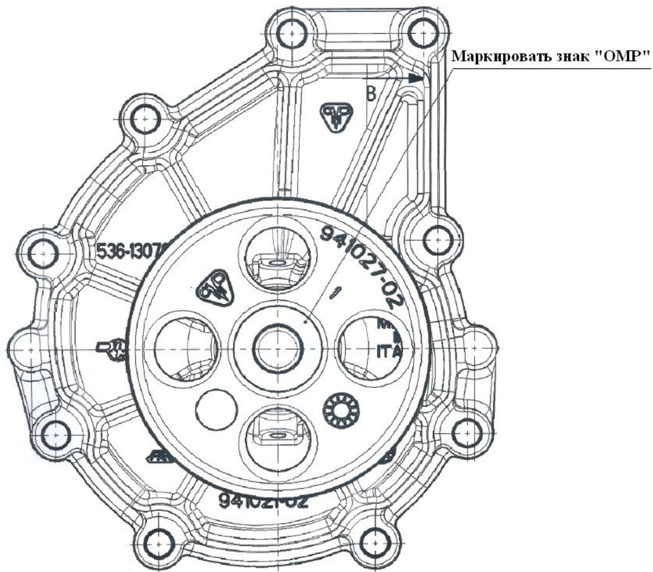
Рис. 2. Водяной насос 536.1307010-20 фирмы «ОМР».
