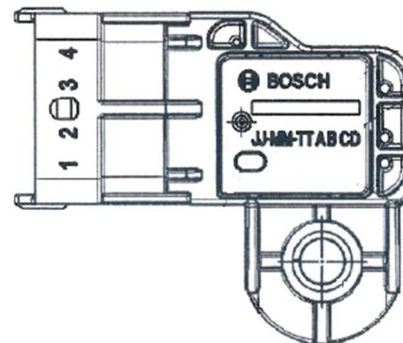
рис. 4. 651.1130548 (BOSCH)
