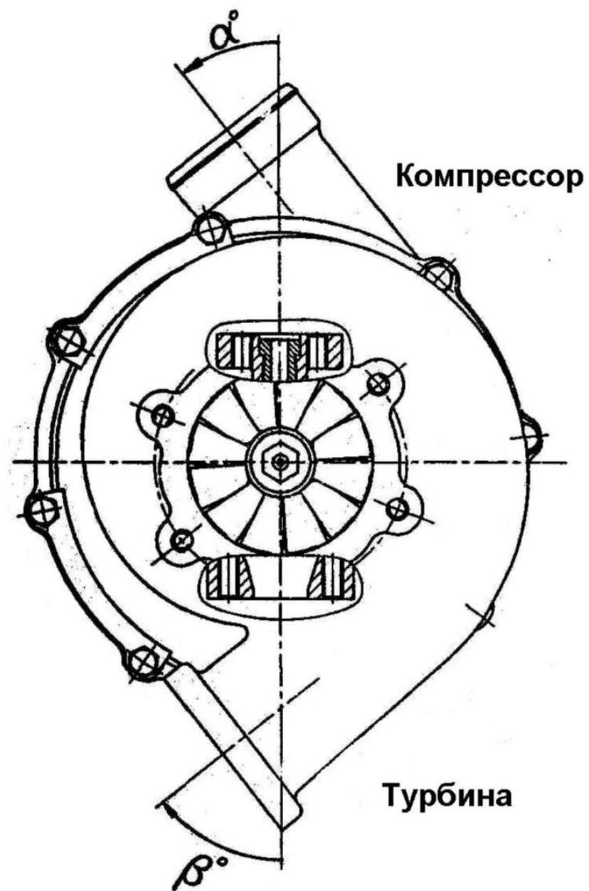
Рисунок 1 – Установка углов разворота турбокомпрессора
