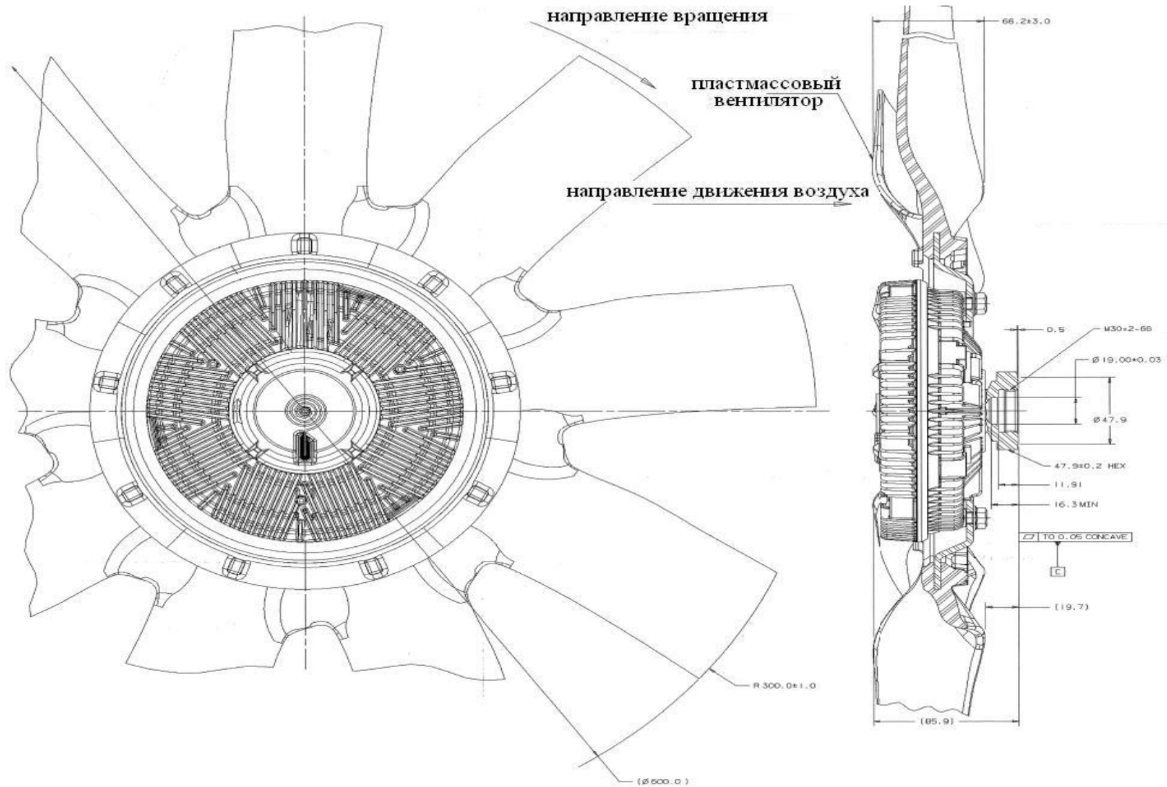
Рисунок 2. Вентилятор "Borg Warner" 020004190.
