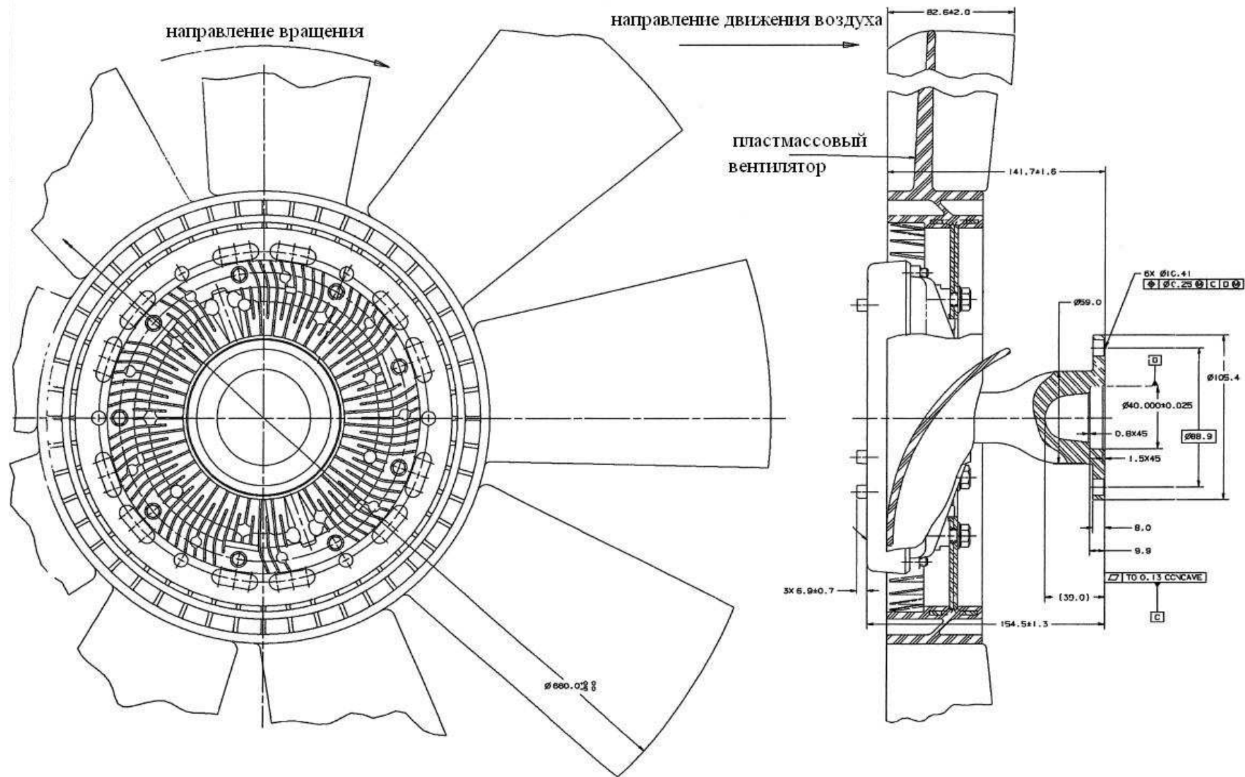
Рисунок 1. Вентилятор “Borg Warner” 020004136.
